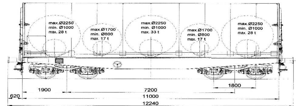
Šema maksimalnog opterećenja kolevki kola serije Shimms
